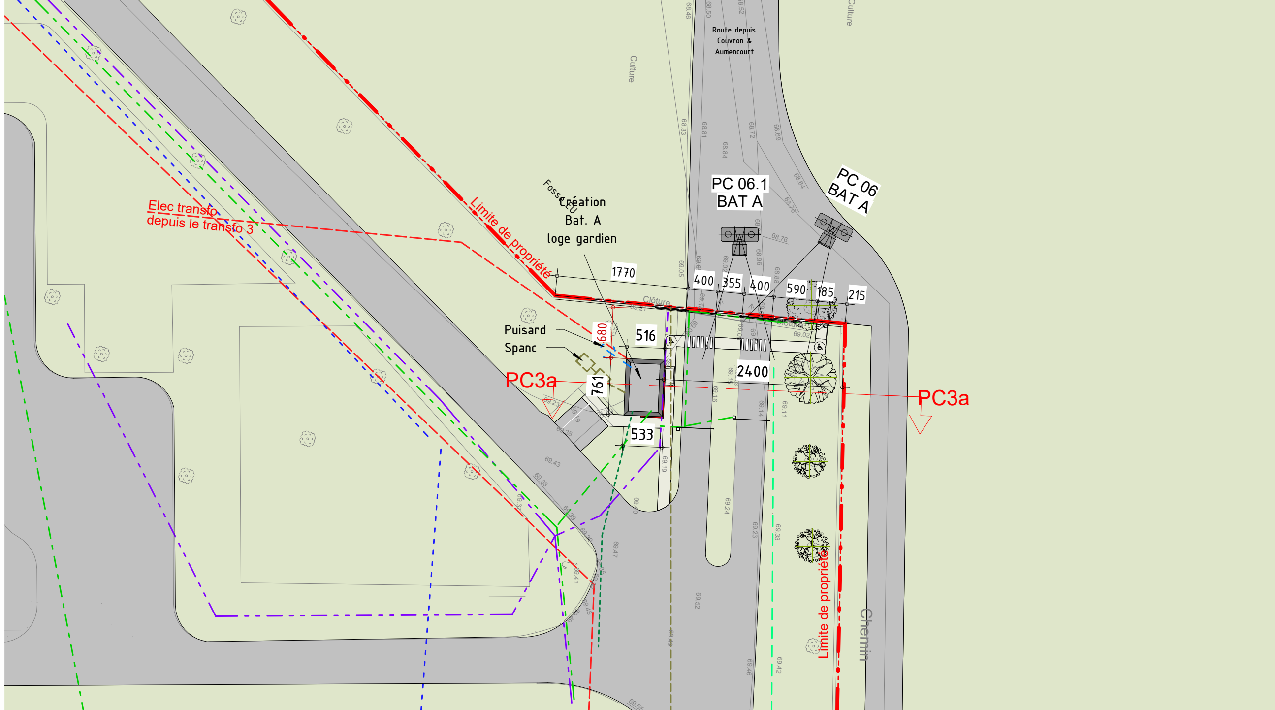
Plan masse PROJET - Zone Loge - ECH : 1 : 500
