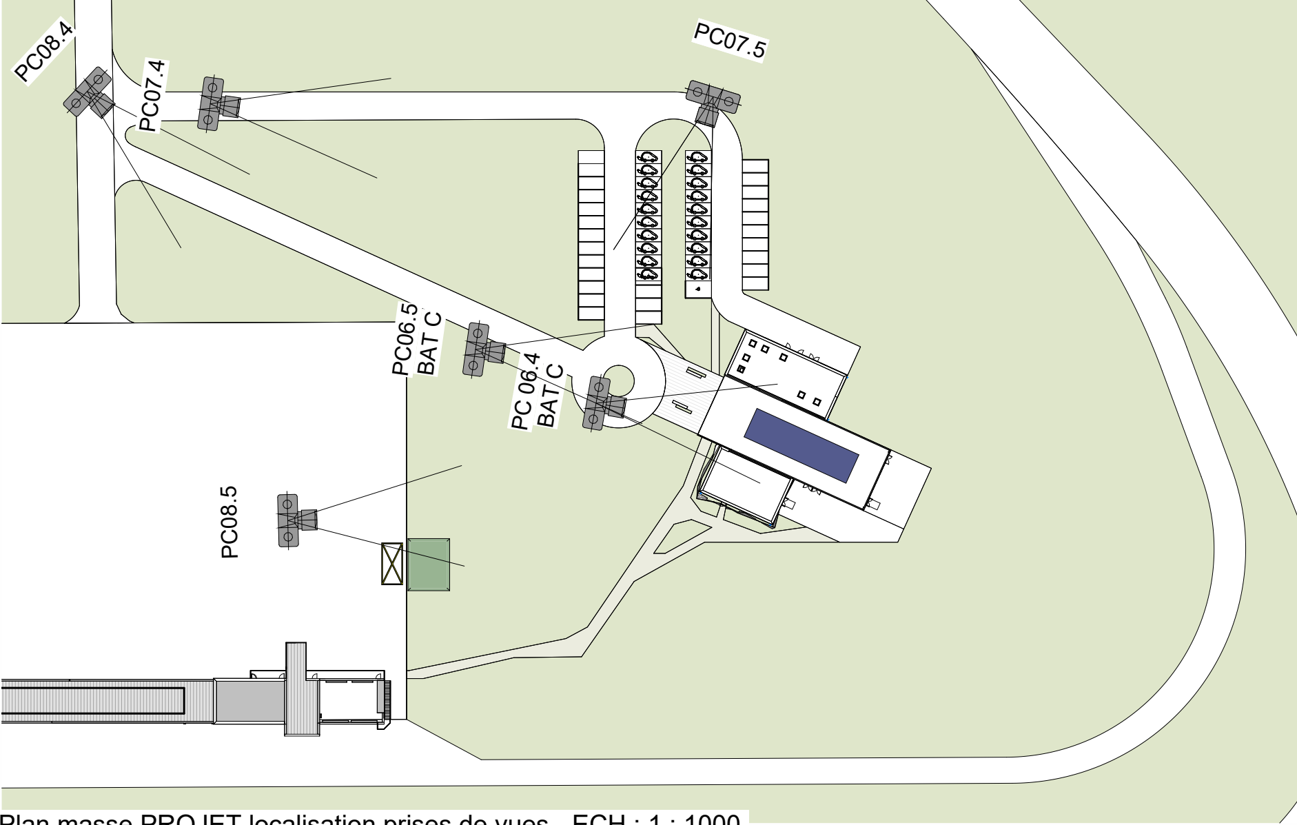
Plan masse PROJET localisation prises de vues - ECH : 1 : 1000
