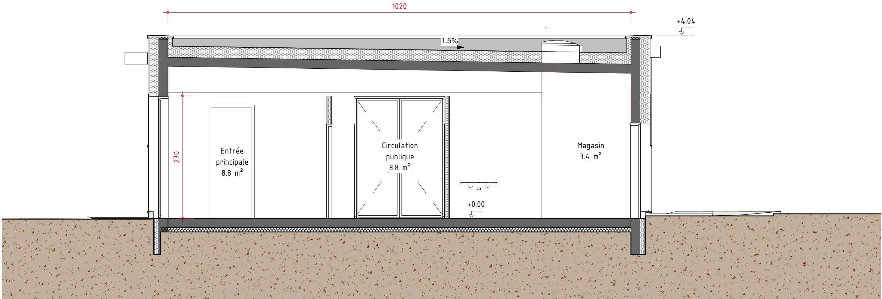
Coupe de principe - ECH : 1 : 50
