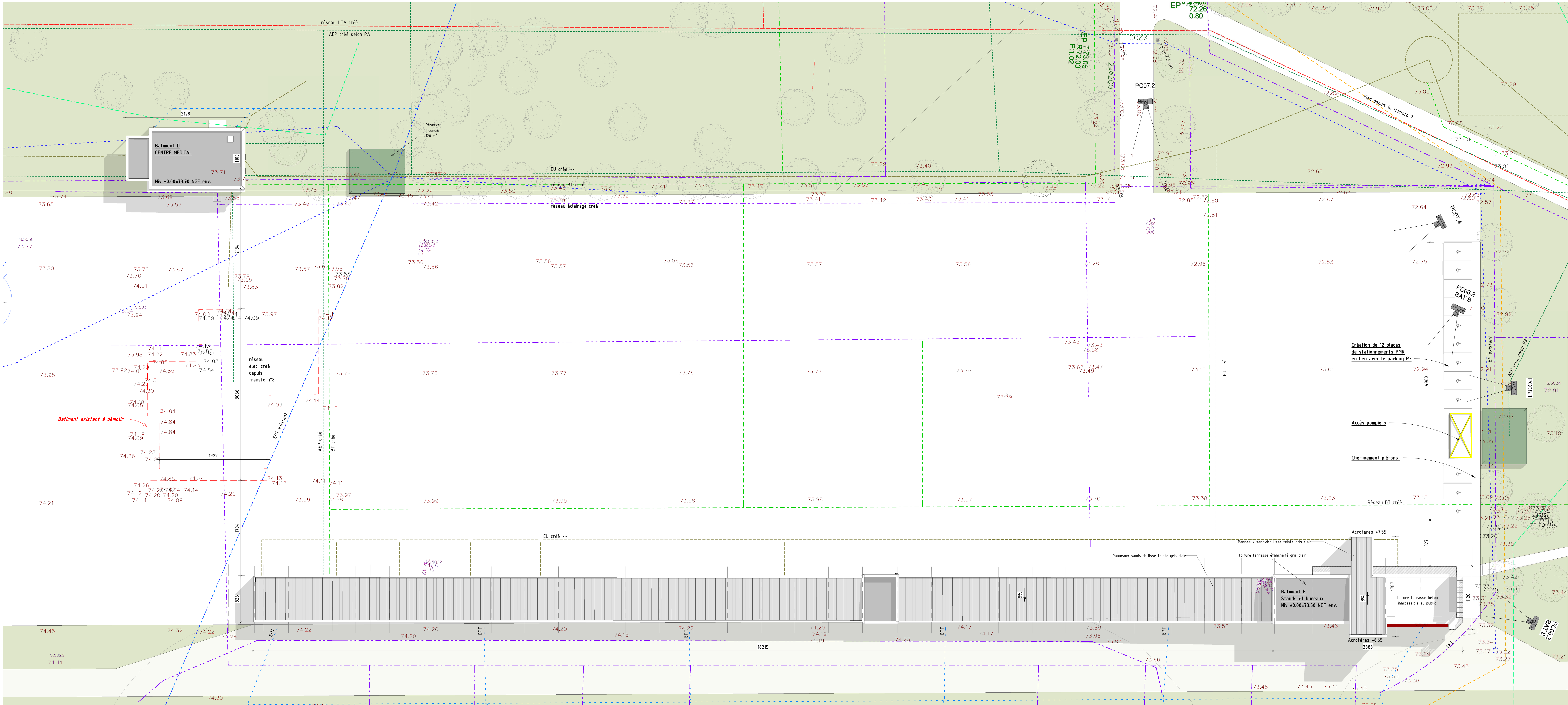
PC05- PLAN DE TOITURE HALL D'EXPOSITIONS - ECH : 1 : 250
