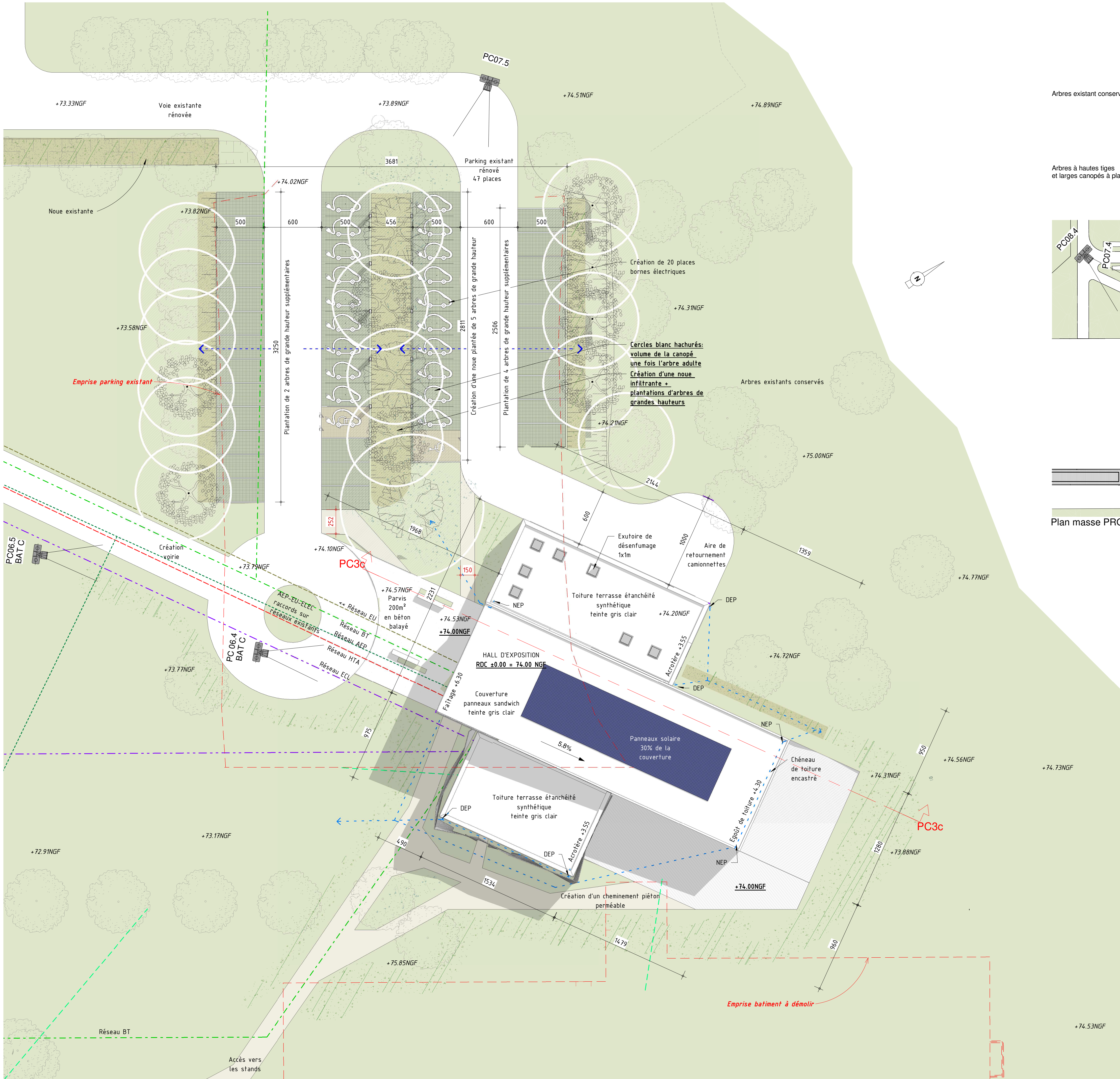
PC02- PLAN DE MASSE PROJET - HALL D'EXPOSITIONS - ECH : 1 : 200
